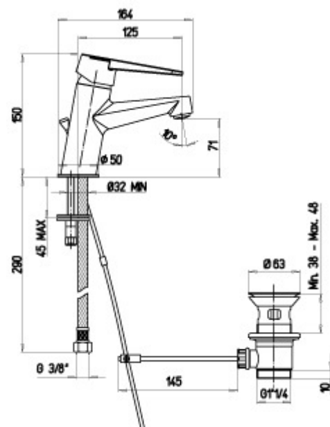
Schéma technique
