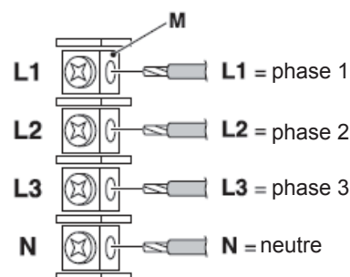
Alimentation 380 V ~
