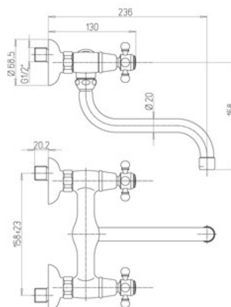
Schéma technique
