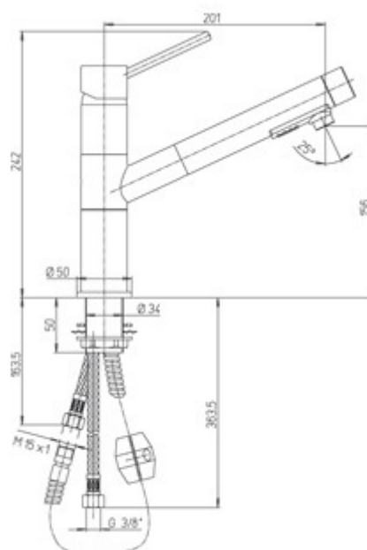
Schéma technique
