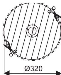
Vasque Uzès S01637 00 xxx (découpe du plan : Ø 320 mm)
